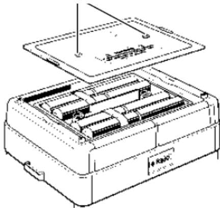
电池盖螺丝
